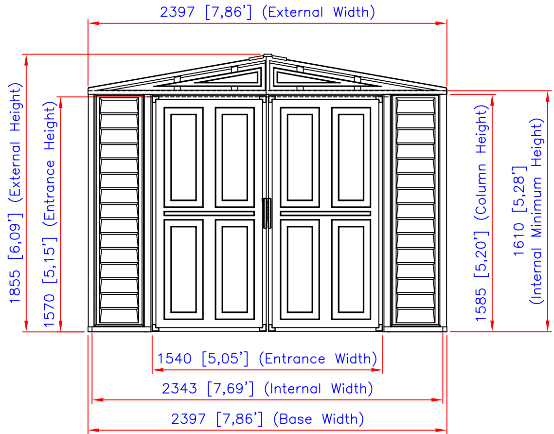
Elevation
